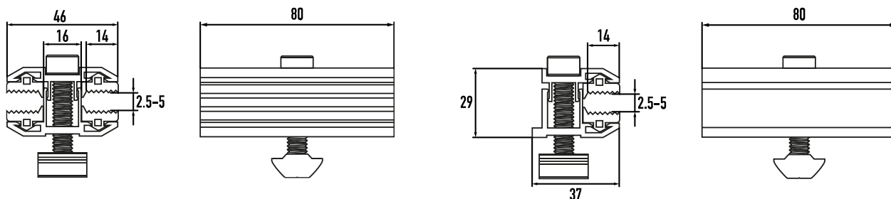
Rys. 11.4.2.2 Przekrój zacisków montażowych: zewnętrzny i wewnętrzny
