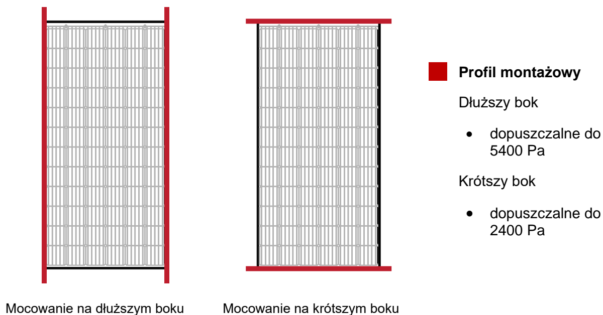
Rys. 11.3.2. Montaż przy użyciu profilu.
