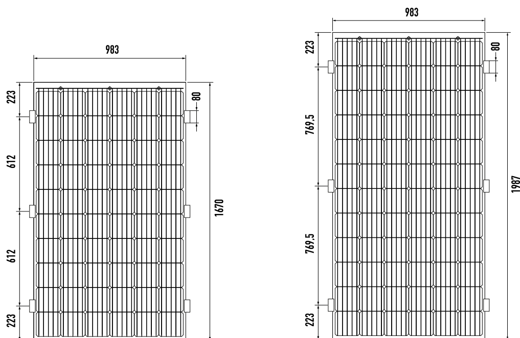
Rys.11.4.2.1 Umieszczenie zacisków montażowych
